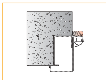
TELAIO E FALSOTELAIO STANDARD CONFORT 15C
