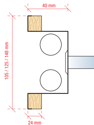
SEZIONE ORIZZONTALE
