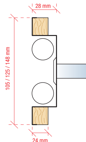
SEZIONE ORIZZONTALE
